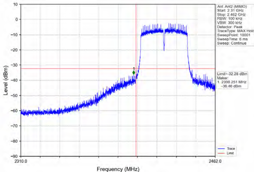
802.11n(HT40)_LCH_2422MHz_Ant2 (MIMO)_NTNV
