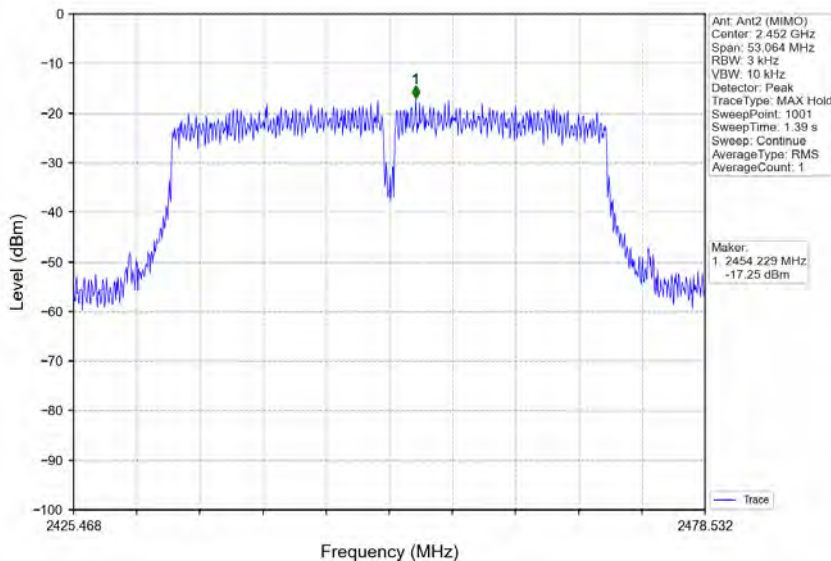
802.11n(HT40)_HCH_2452MHz_MIMO_NTNV
