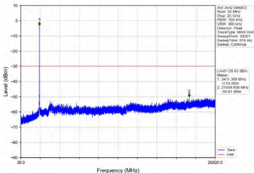
802.11n(HT20)_LCH_2412MHz_Ant2 (MIMO)_NTNV
