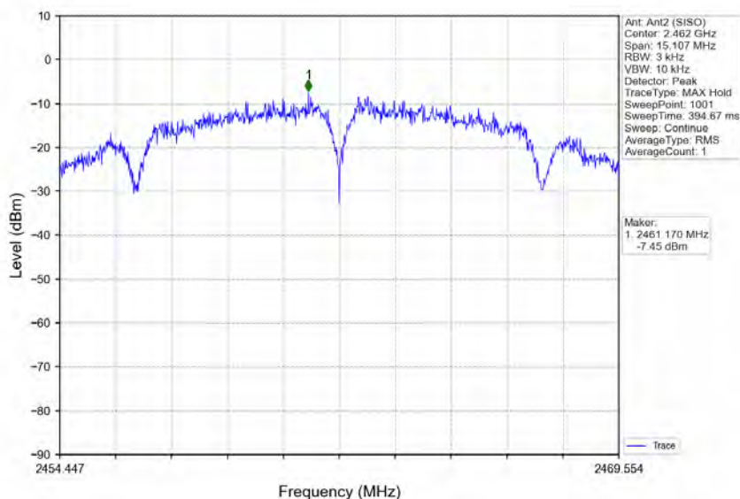
802.11b_HCH_2462MHz_Ant2 (SISO)_NTNV
