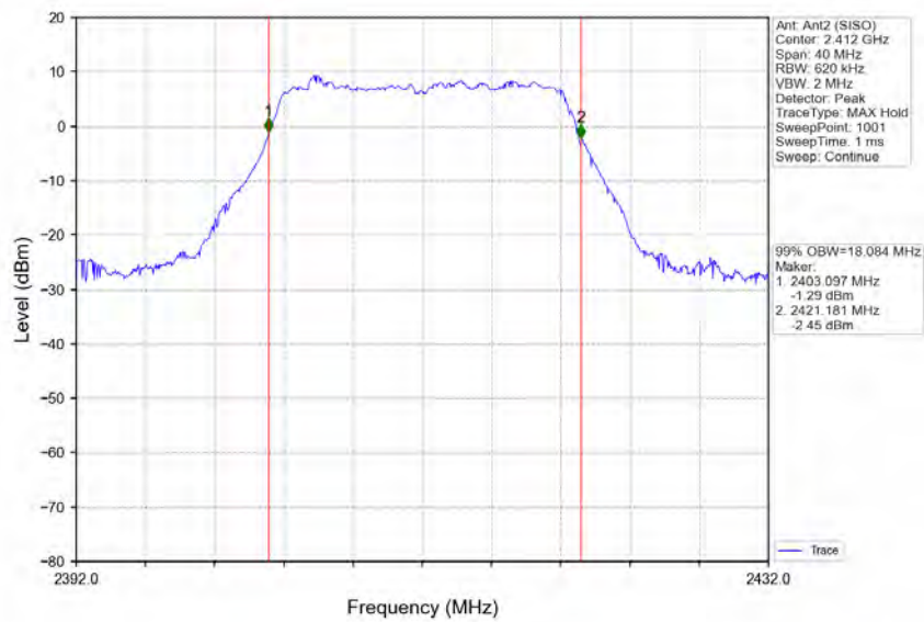
802.11g_LCH_2412MHz_Ant2 (SISO)_NTNV
