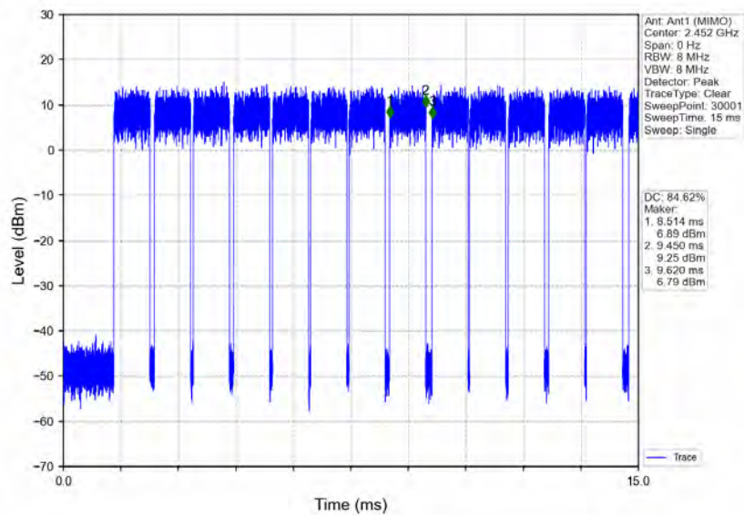
802.11n(HT40)_HCH_2452MHz_Ant1 (MIMO)_NTNV
