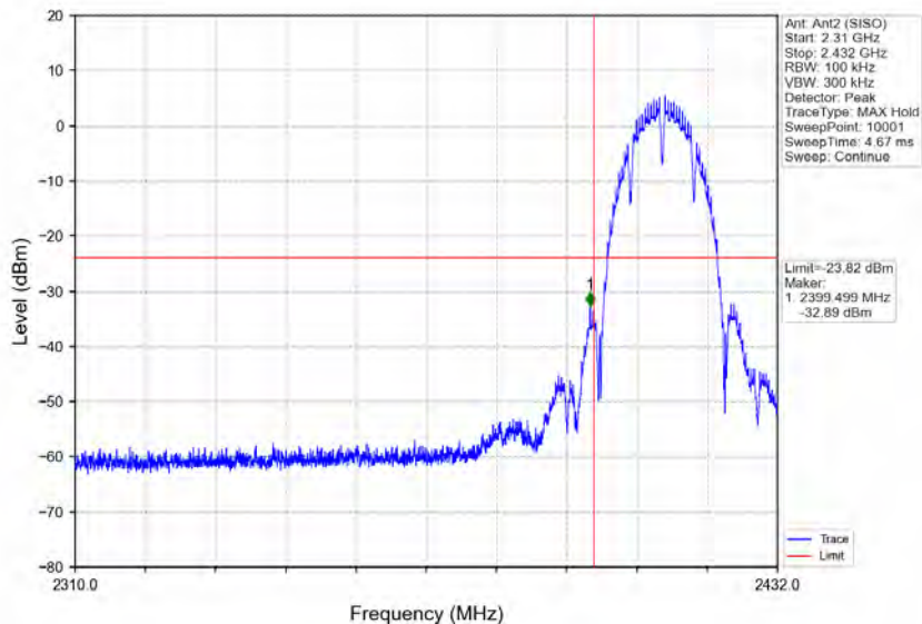
802.11b_LCH_2412MHz_Ant2 (SISO)_NTNV
