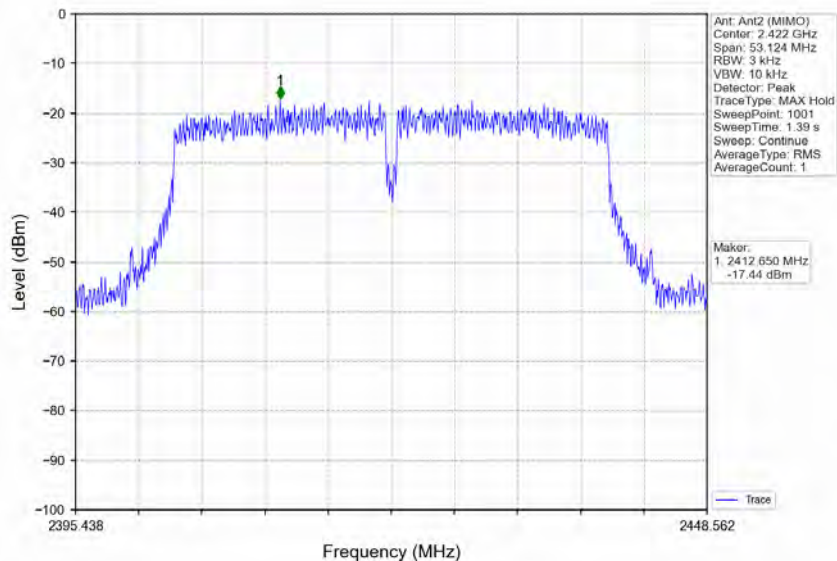
802.11n(HT40)_LCH_2422MHz_MIMO_NTNV
