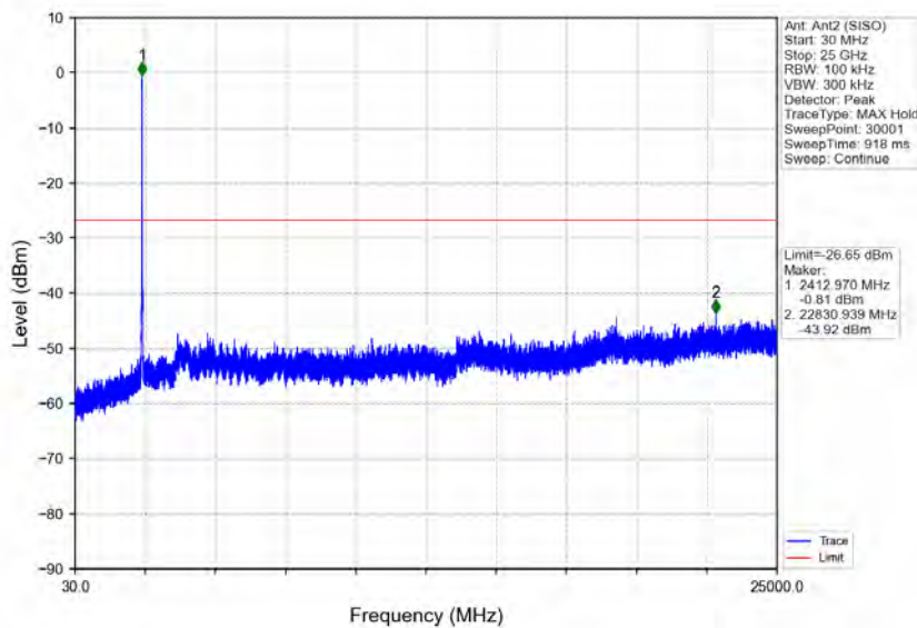
802.11g_LCH_2412MHz_Ant2 (SISO)_NTNV
