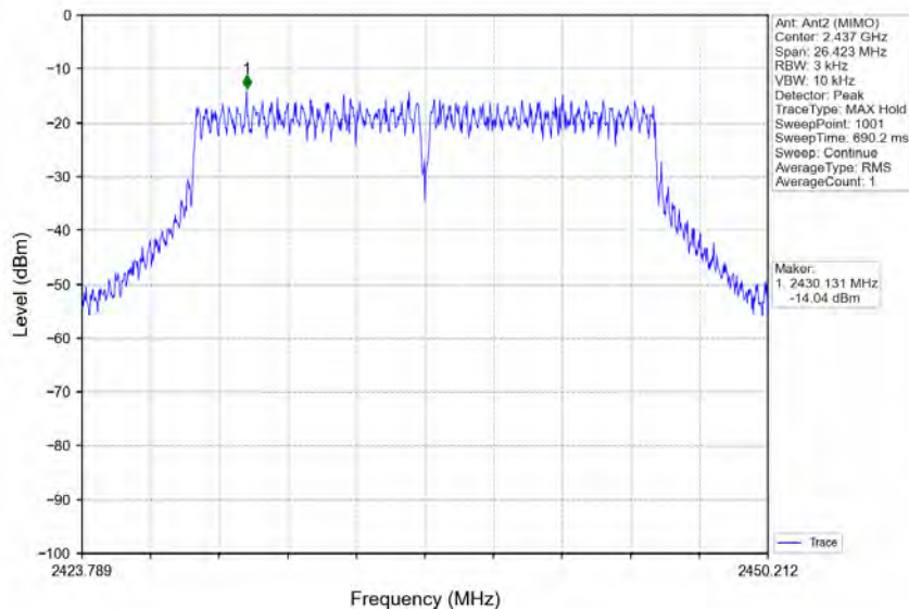
802.11n(HT20)_MCH_2437MHz_MIMO_NTNV
