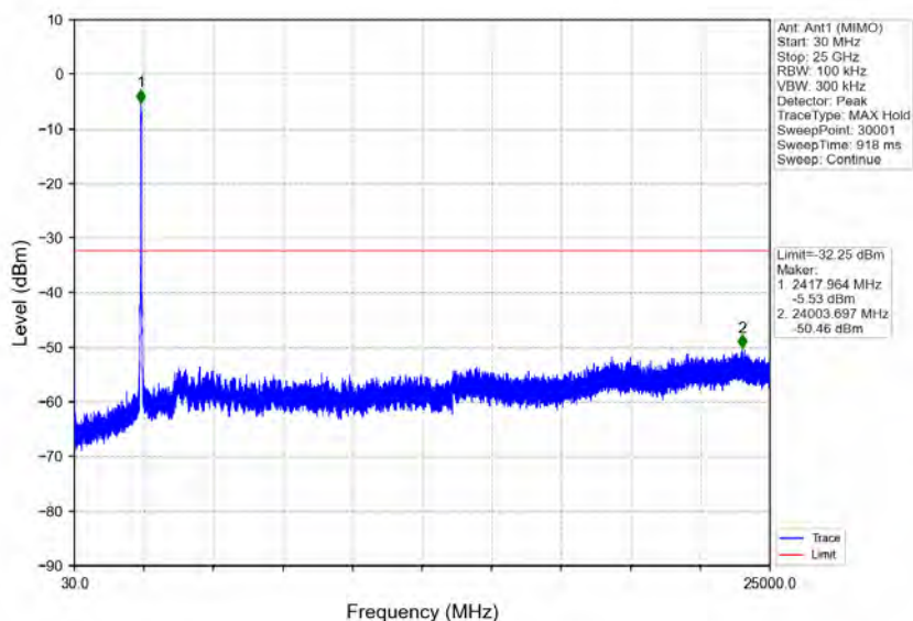
802.11n(HT40)_LCH_2422MHz_Ant1 (MIMO)_NTNV
