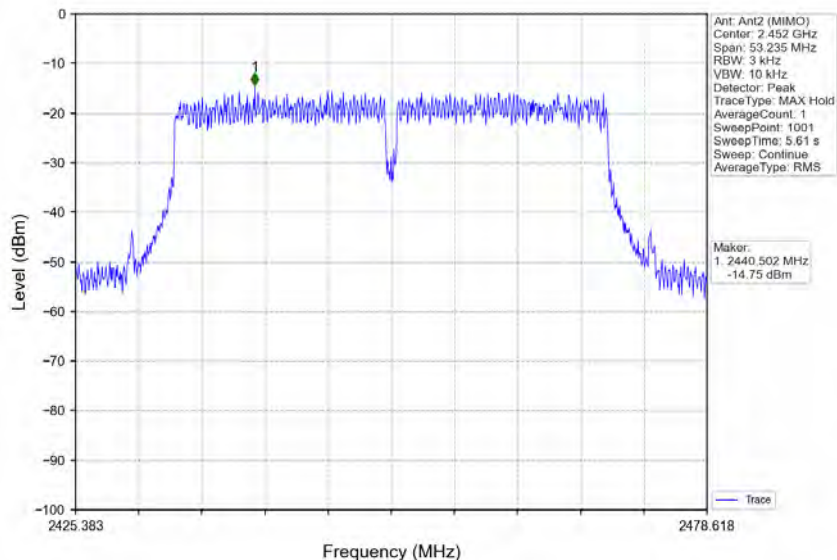
802.11n(HT40)_HCH_2452MHz_MIMO_NTNV
