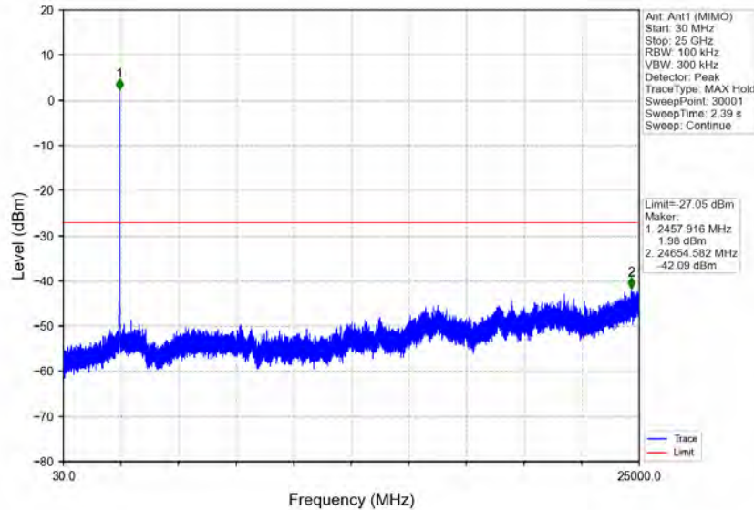
802.11n(HT20)_HCH_2462MHz_Ant1 (MIMO)_NTNV
