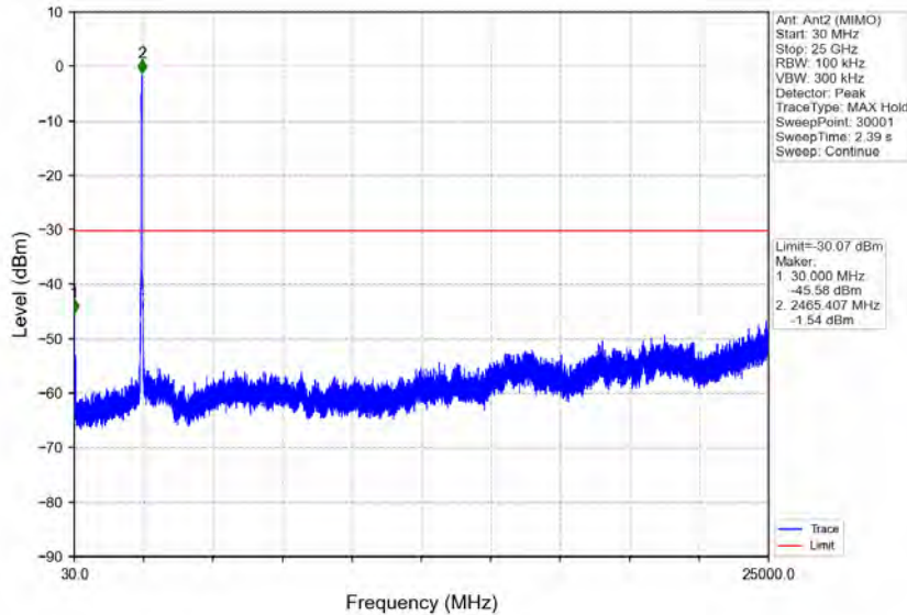
802.11n(HT40)_HCH_2452MHz_Ant2 (MIMO)_NTNV
