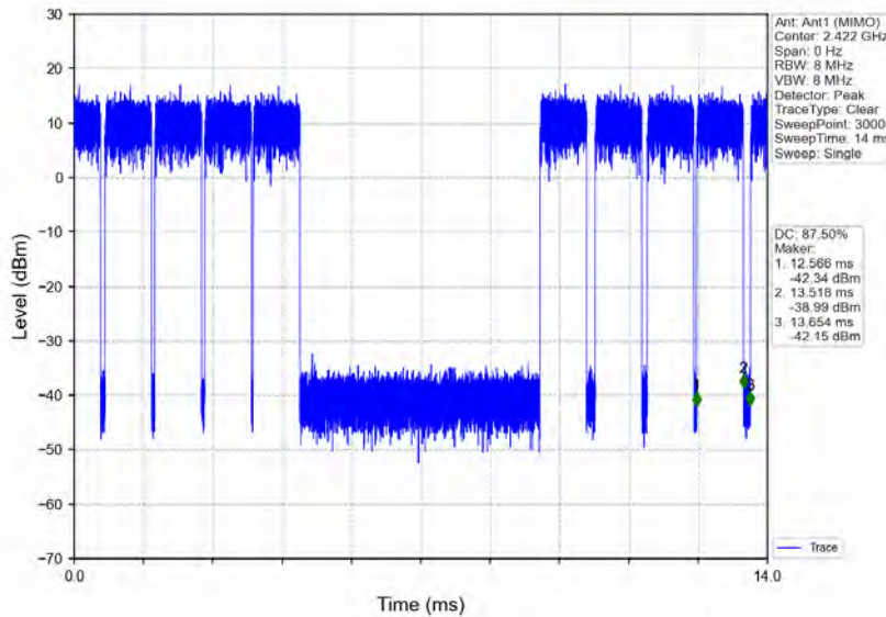
802.11n(HT40)_LCH_2422MHz_Ant1 (MIMO)_NTNV
