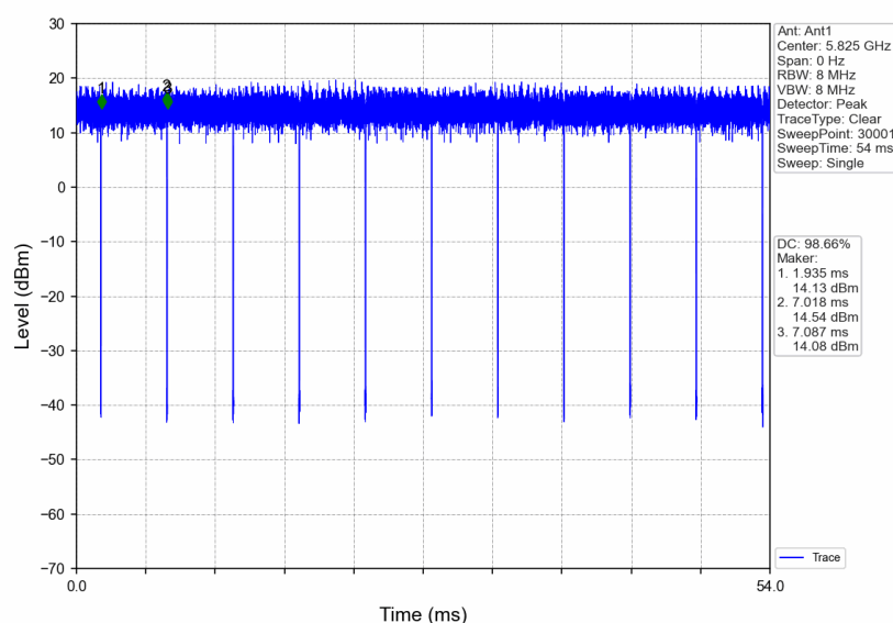
802.11n(HT20)_HCH_5825MHz_Ant1_NTNV
