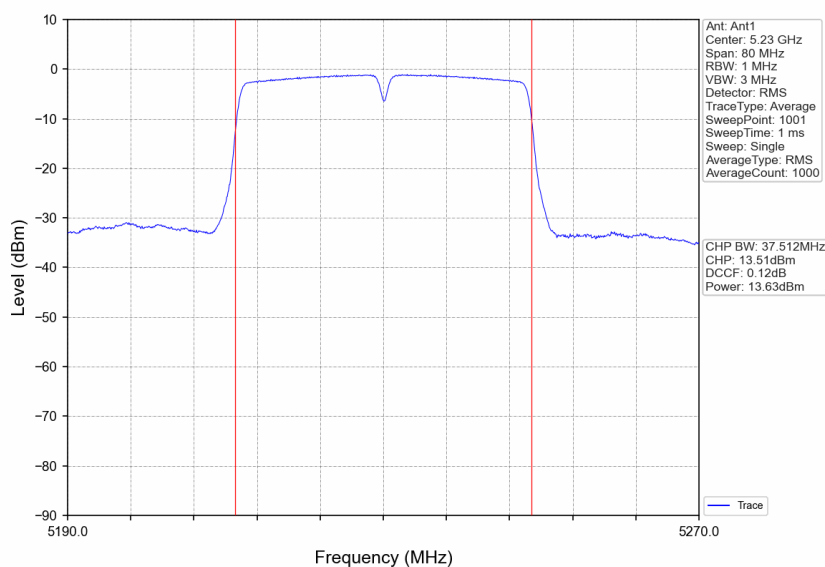
802.11n(HT40)_HCH_5230MHz_Ant1_NTNV
