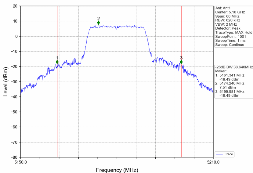
802.11n(HT20)_LCH_5180MHz_Ant1_NTNV
