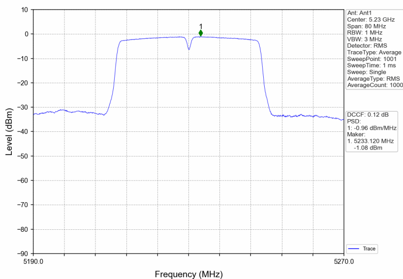
802.11n(HT40)_HCH_5230MHz_Ant1_NTNV
