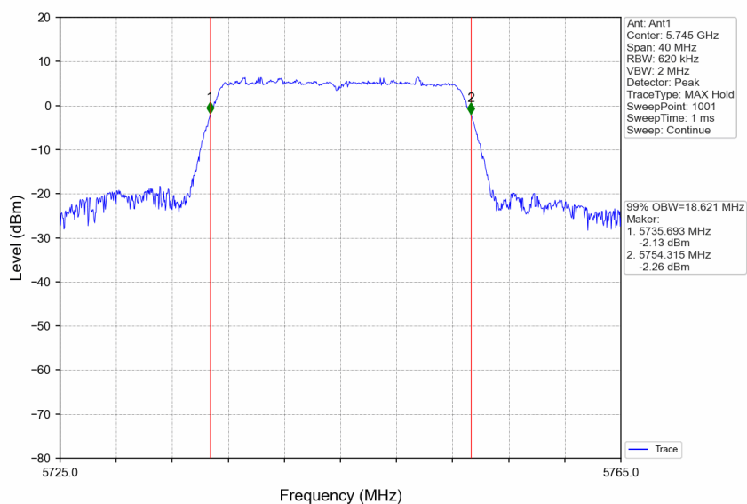
802.11n(HT20)_LCH_5745MHz_Ant1_NTNV
