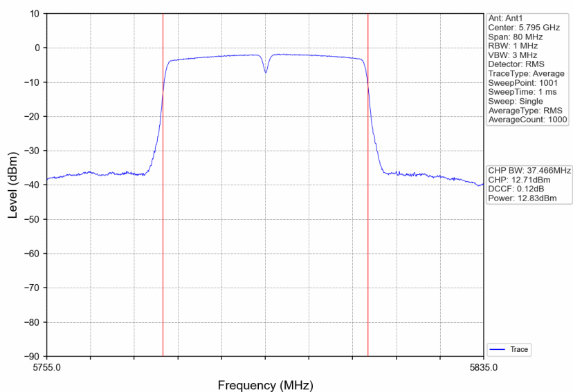
802.11n(HT40)_HCH_5795MHz_Ant1_NTNV
