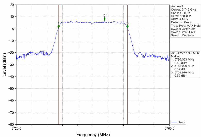
802.11n(HT20)_LCH_5745MHz_Ant1_NTNV
