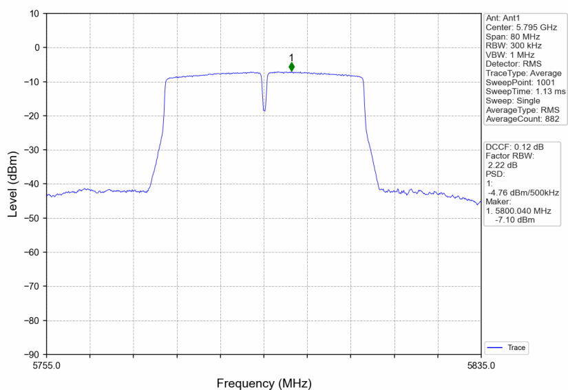
802.11n(HT40)_HCH_5795MHz_Ant1_NTNV
