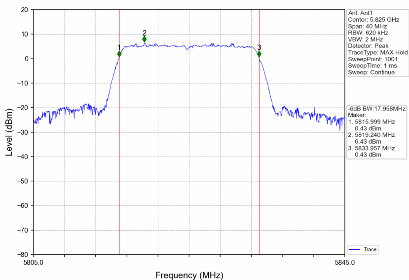
802.11n(HT20)_HCH_5825MHz_Ant1_NTNV
