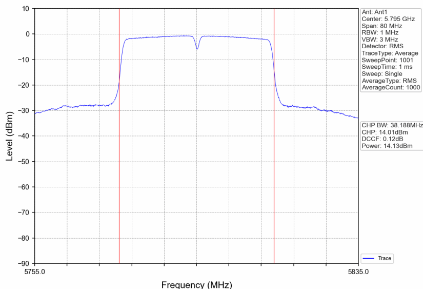
802.11n(HT40)_HCH_5795MHz_Ant1_NTNV
