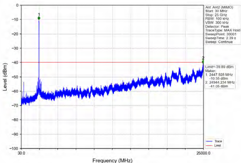
802.11n(HT40)_HCH_2452MHz_Ant2 (MIMO)_NTNV
