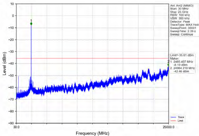
802.11n(HT20)_HCH_2462MHz_Ant2 (MIMO)_NTNV
