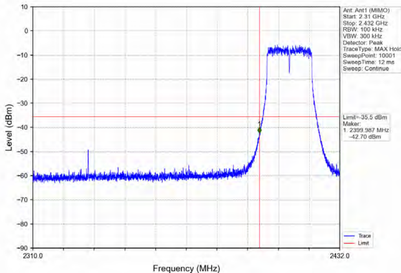
802.11n(HT20)_LCH_2412MHz_Ant1 (MIMO)_NTNV
