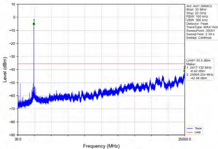
802.11n(HT20)_LCH_2412MHz_Ant1 (MIMO)_NTNV
