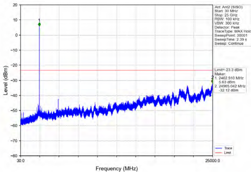
802.11b_HCH_2462MHz_Ant2 (SISO)_NTNV
