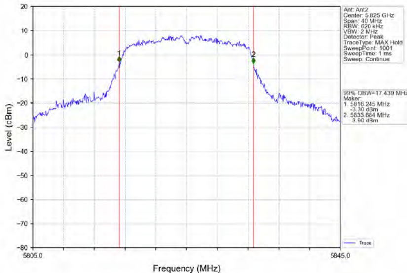
802.11a_HCH_5825MHz_Ant2_NTNV
