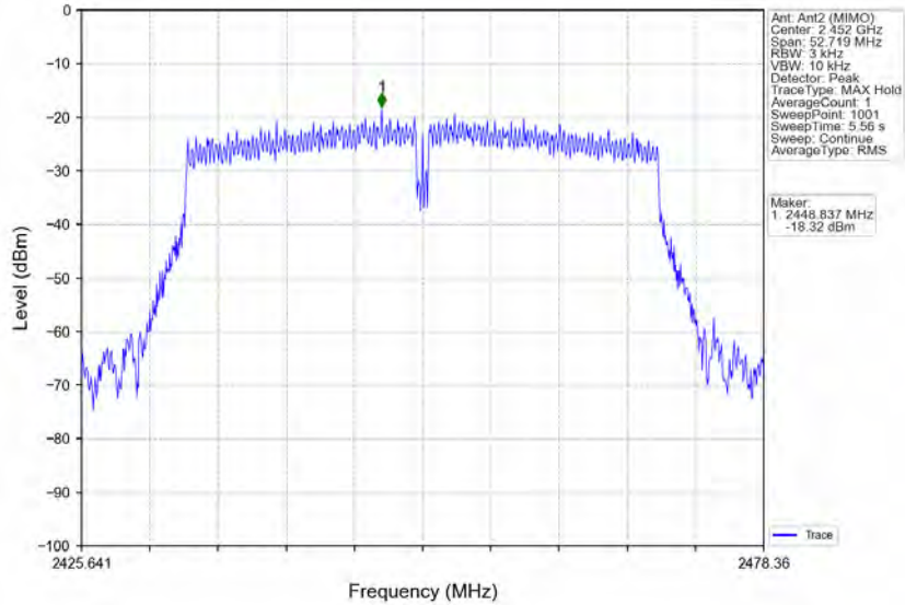
802.11n(HT40)_HCH_2452MHz_MIMO_NTNV
