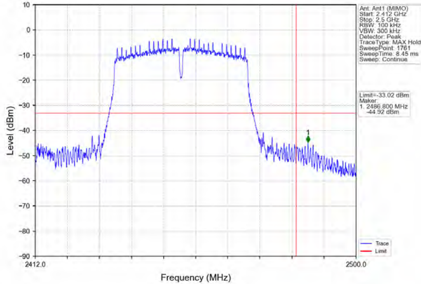
802.11n(HT40)_HCH_2452MHz_Ant1 (MIMO)_NTNV
