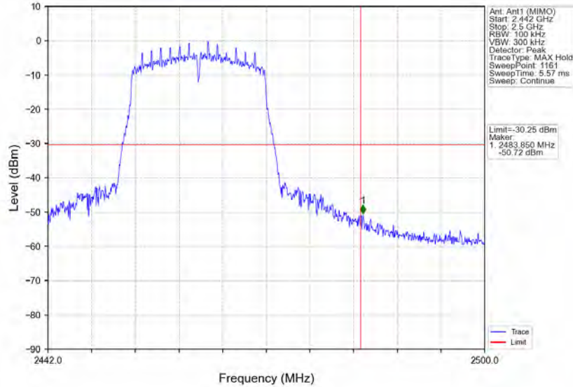
802.11n(HT20)_HCH_2462MHz_Ant1 (MIMO)_NTNV
