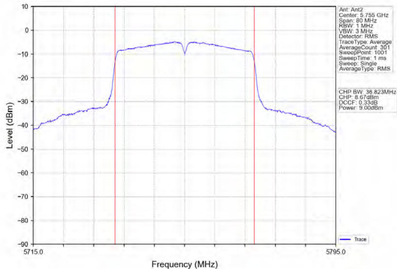
802.11ac(VHT40)_LCH_5755MHz_Ant2_NTNV
