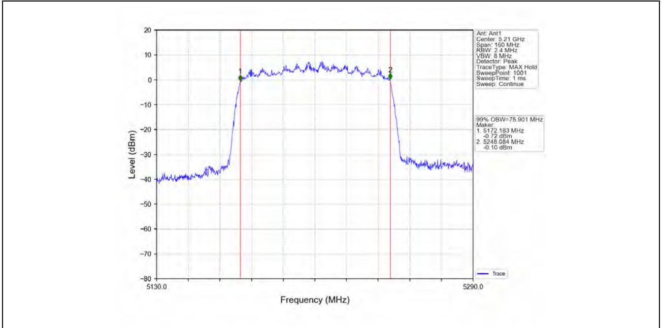
802.11ac(VHT80)_MCH_5210MHz_Ant2_NTNV
