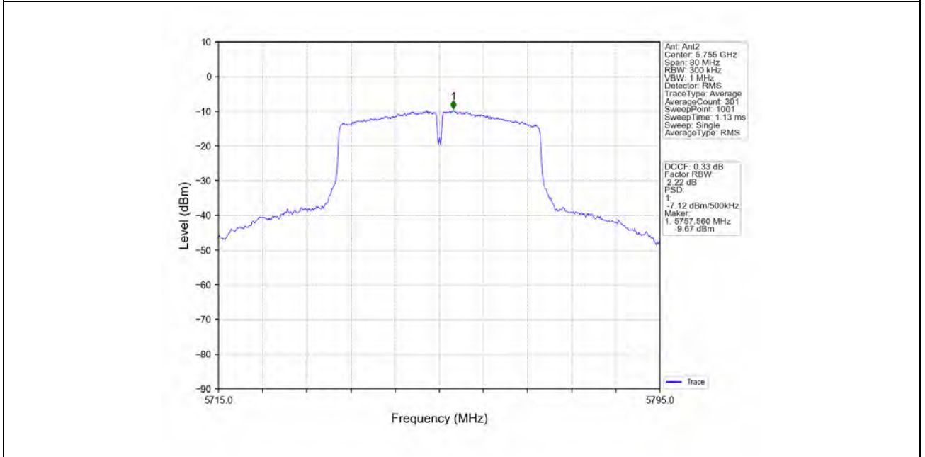
802.11ac(VHT40)_LCH_5755MHz_MIMO_NTNV
