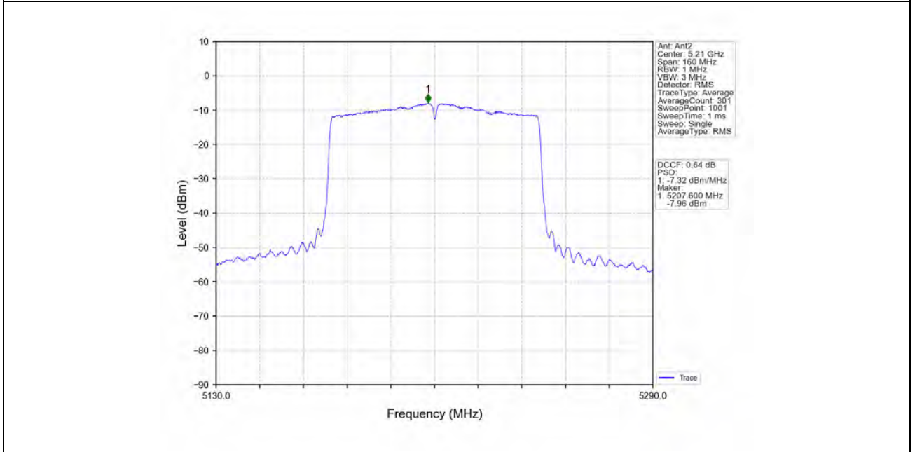
802.11ac(VHT80)_MCH_5210MHz_MIMO_NTNV
