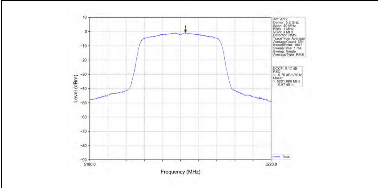
802.11n(HT20)_MCH_5200MHz_MIMO_NTNV
