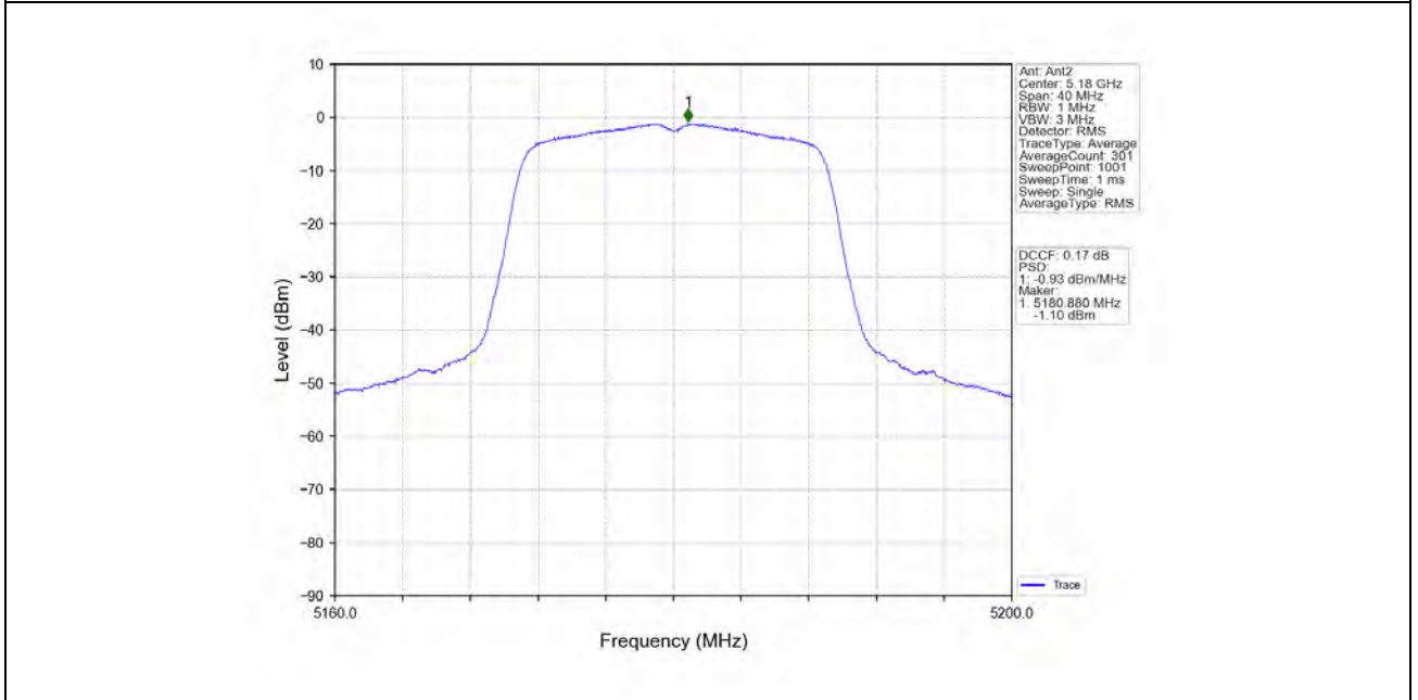
802.11n(HT20)_LCH_5180MHz_MIMO_NTNV
