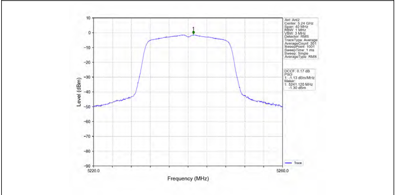
802.11n(HT20)_HCH_5240MHz_MIMO_NTNV
