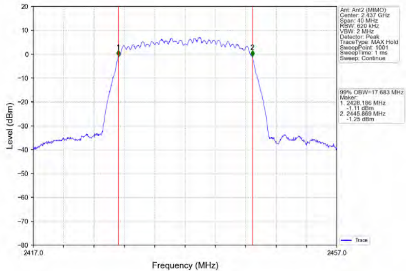
802.11n(HT20)_MCH_2437MHz_Ant2 (MIMO)_NTNV
