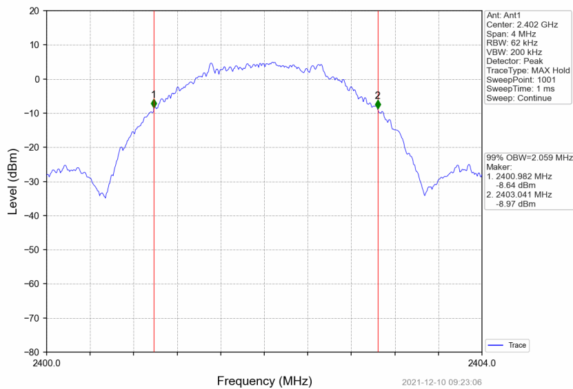
2M_LCH_2402MHz_DataRate=_Ant1_NTNV
