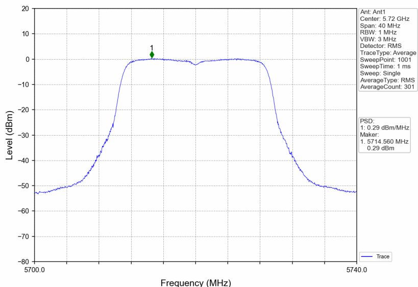
802.11ac(VHT20)_HCH_5720MHz_Ant1_NTNV
