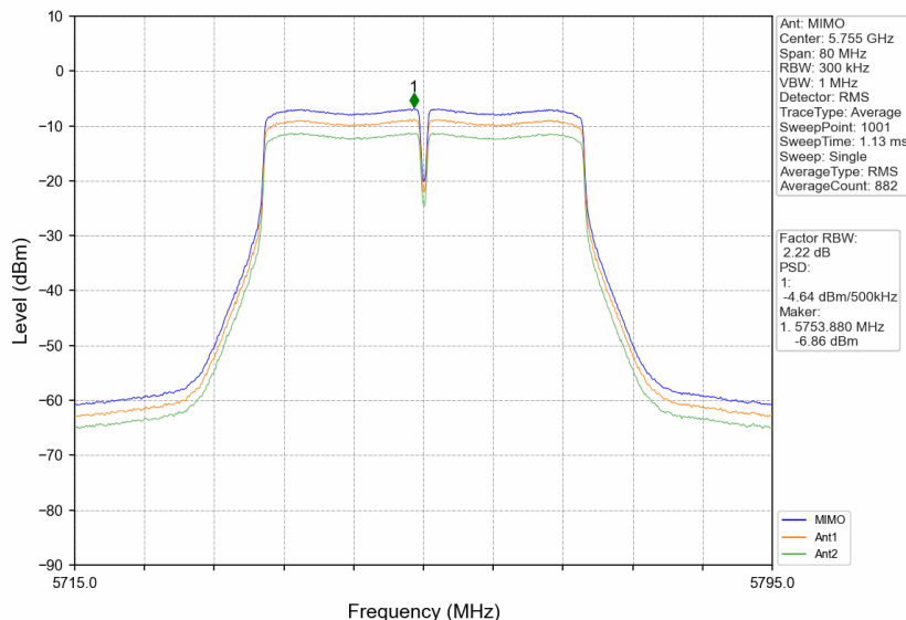
802.11n(HT40)_LCH_5755MHz_MIMO_NTNV
