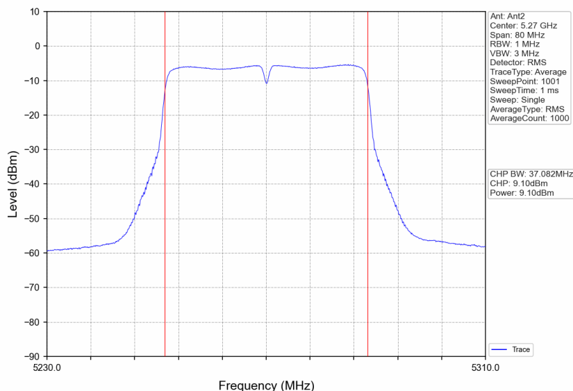
802.11n(HT40)_LCH_5270MHz_Ant2_NTNV
