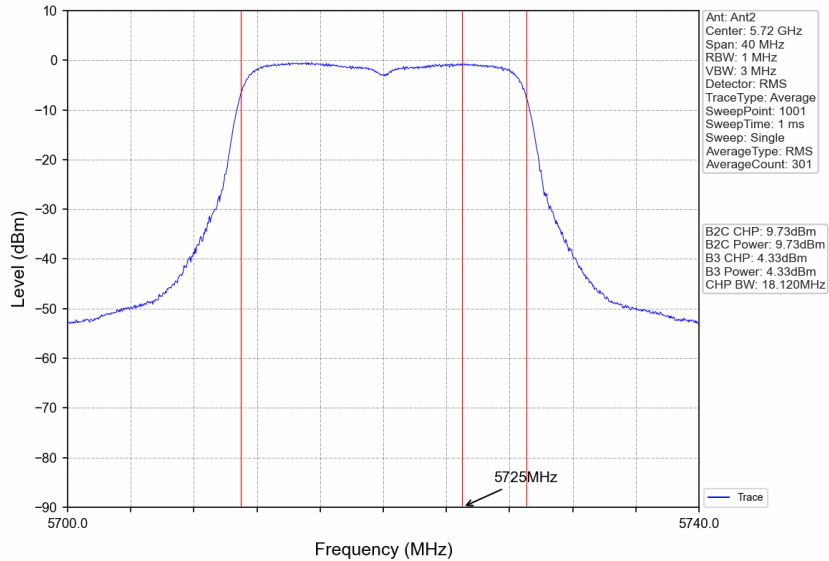
802.11n(HT20)_HCH_5720MHz_Ant2_NTNV
