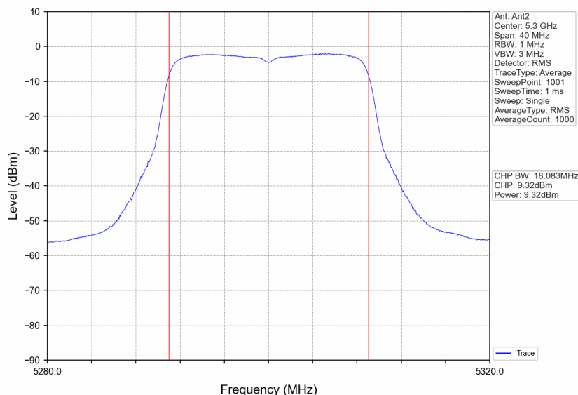
802.11n(HT20)_MCH_5300MHz_Ant2_NTNV
