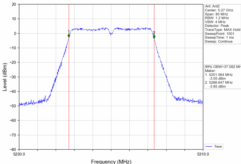
802.11n(HT40)_LCH_5270MHz_Ant2_NTNV
