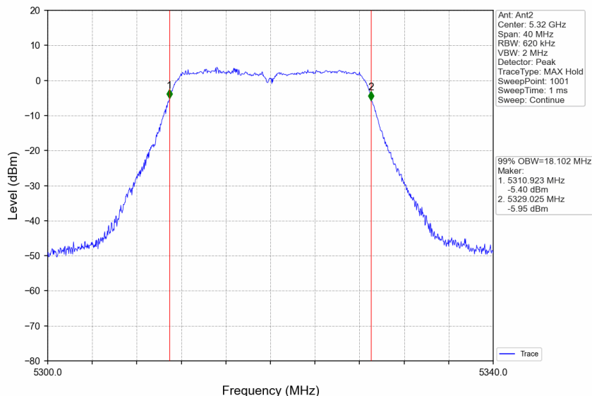
802.11n(HT20)_HCH_5320MHz_Ant2_NTNV
