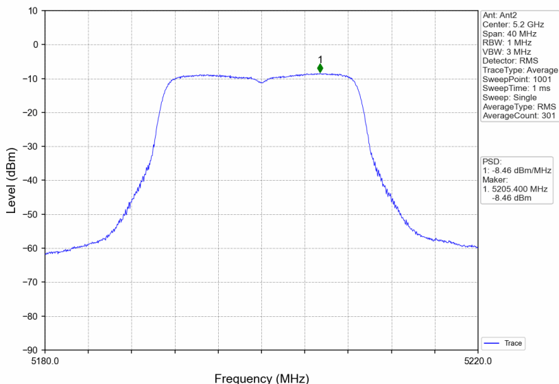
802.11n(HT20)_MCH_5200MHz_MIMO_NTNV
