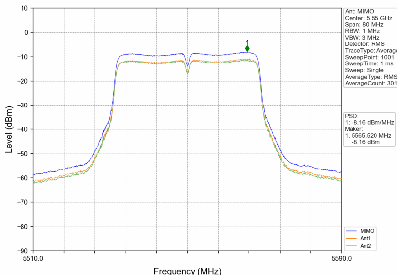
802.11n(HT40)_MCH_5550MHz_MIMO_NTNV
