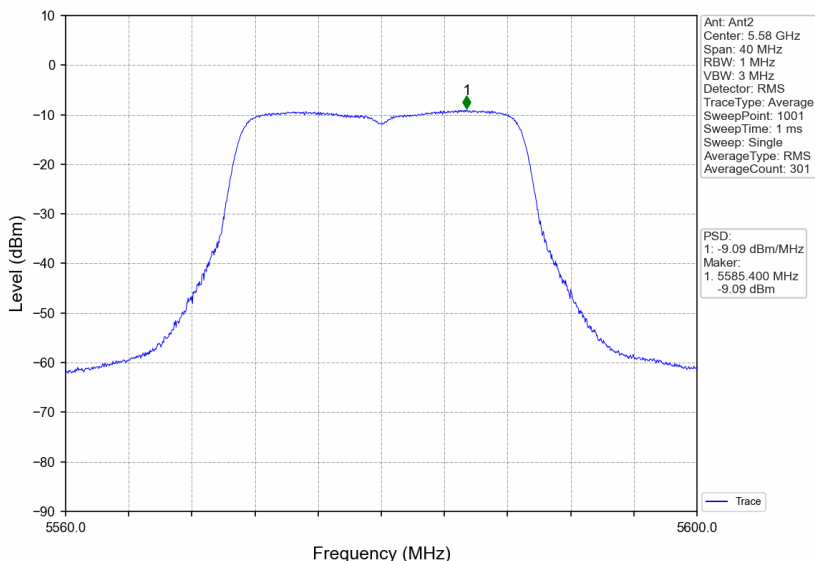
802.11n(HT20)_MCH_5580MHz_MIMO_NTNV
