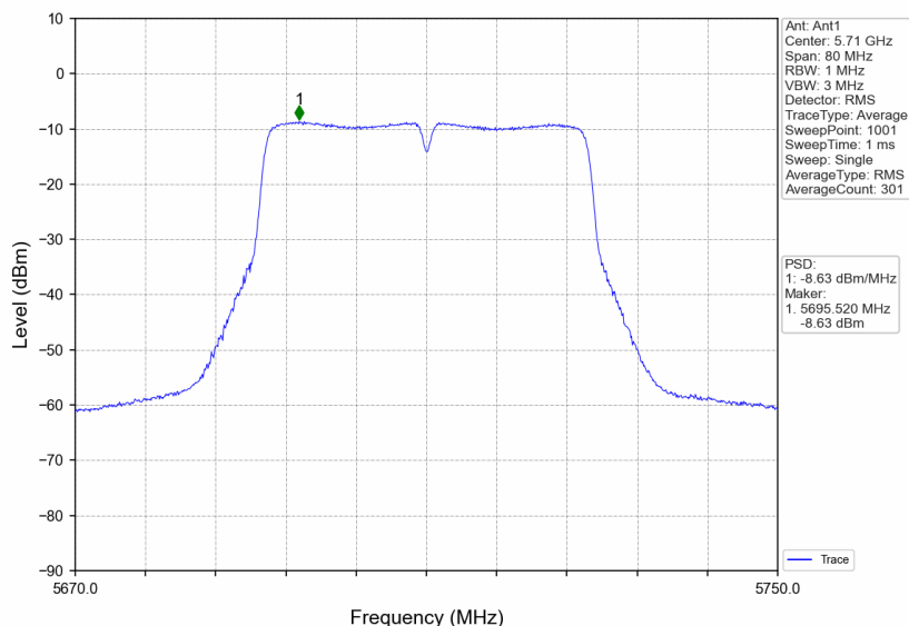
802.11n(HT40)_HCH_5710MHz_Ant1_NTNV
