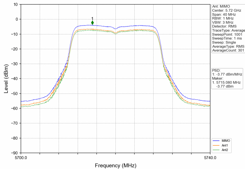
802.11n(HT20)_HCH_5720MHz_MIMO_NTNV
