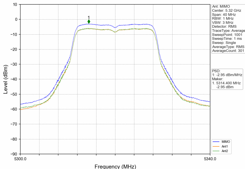
802.11n(HT20)_HCH_5320MHz_MIMO_NTNV
