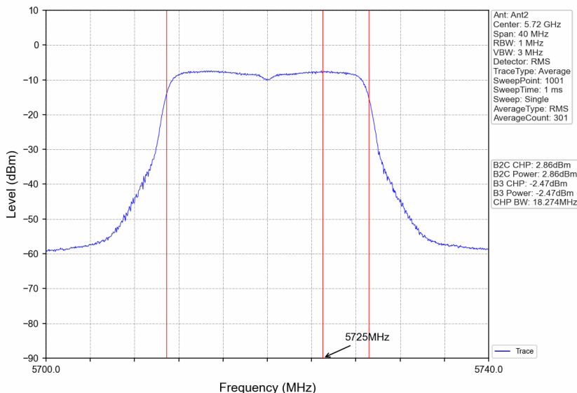
802.11ac(VHT20)_HCH_5720MHz_Ant2_NTNV
