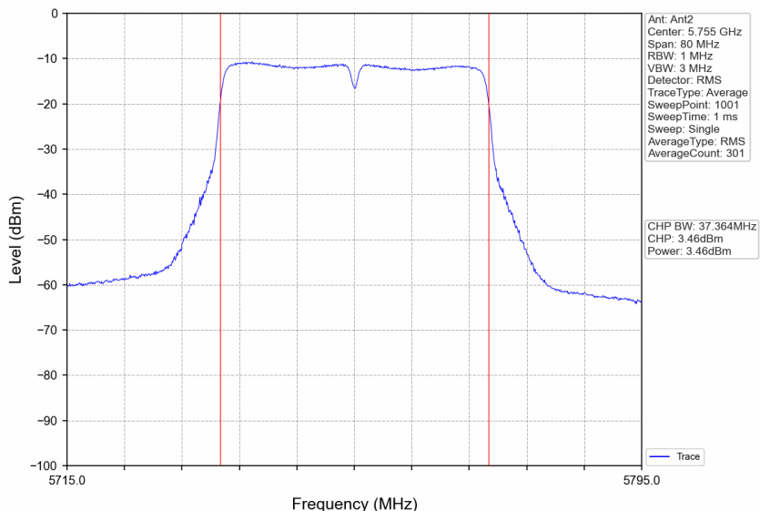
802.11n(HT40)_LCH_5755MHz_Ant2_NTNV
