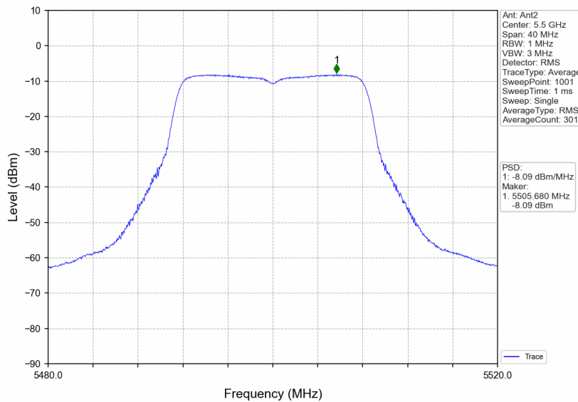
802.11a_LCH_5500MHz_Ant2_NTNV
