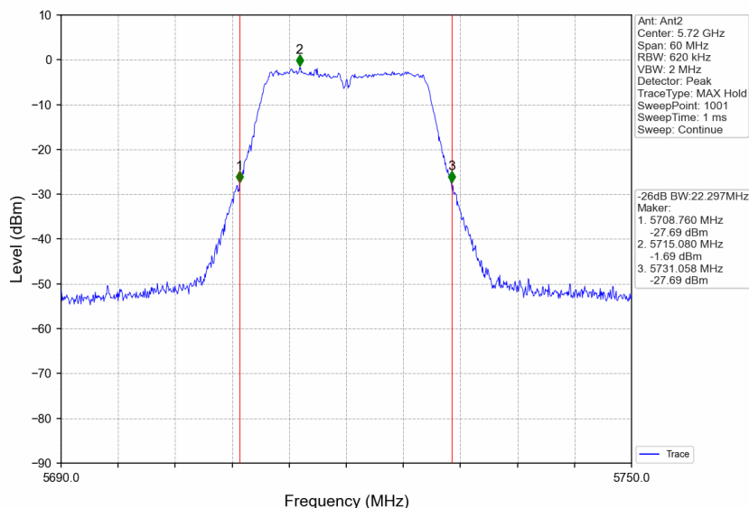
802.11n(HT20)_HCH_5720MHz_Ant2_NTNV
