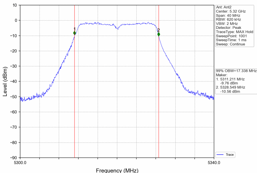
802.11a_HCH_5320MHz_Ant2_NTNV
