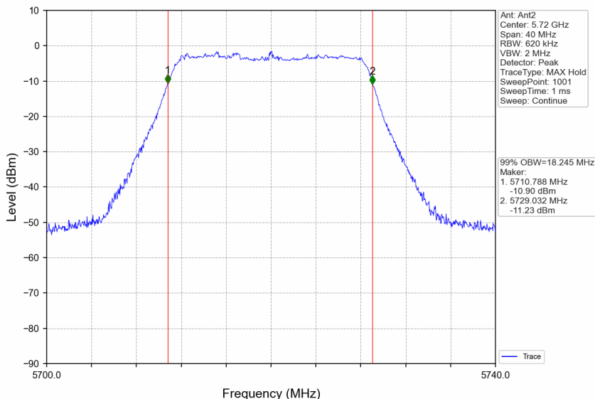
802.11n(HT20)_HCH_5720MHz_Ant2_NTNV
