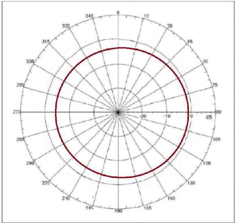
2450MHz
