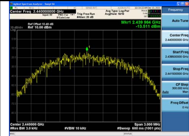
Test Mode:GFSK (LE 2Mbps) MHz
