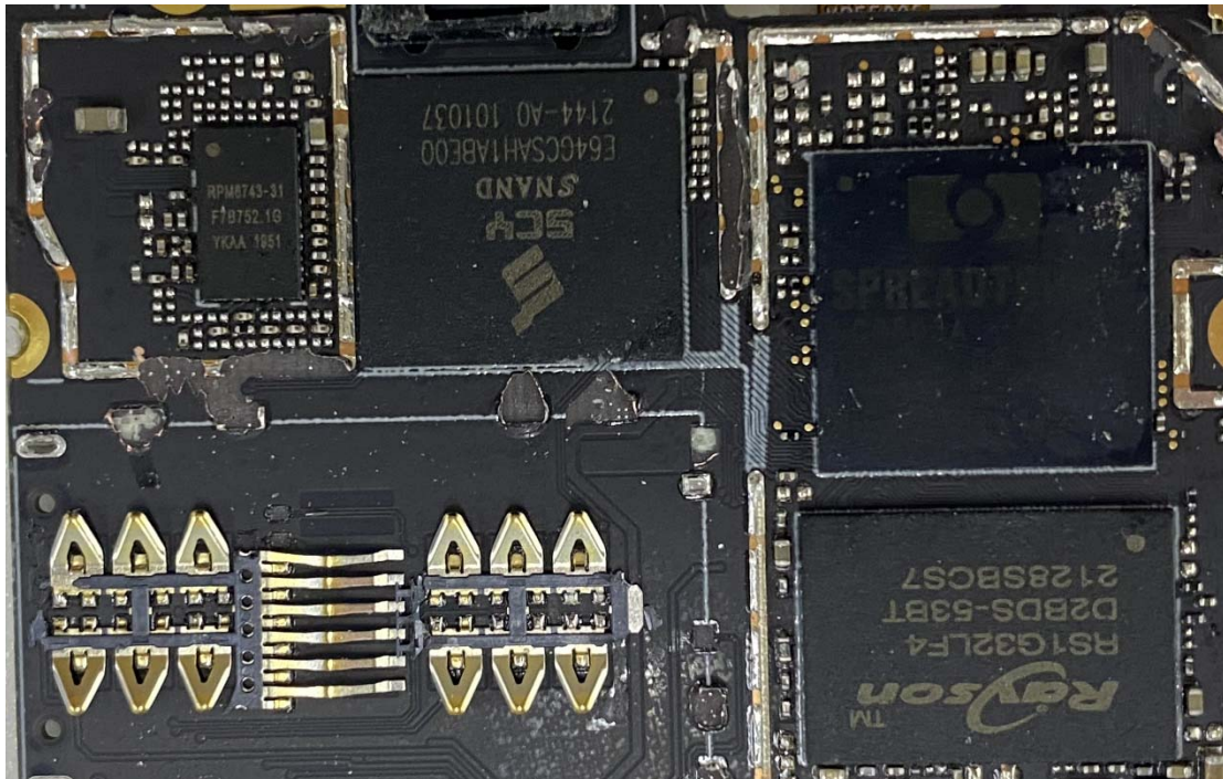
IC Details 4
