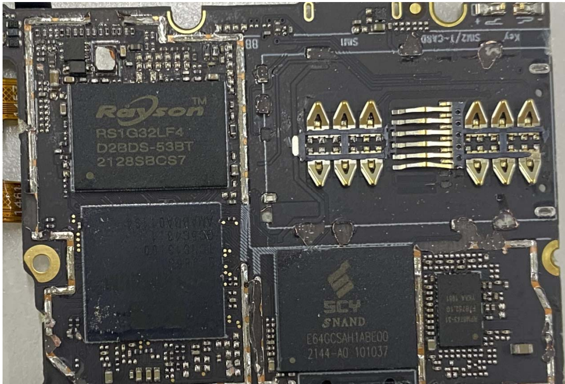
IC Details 3
