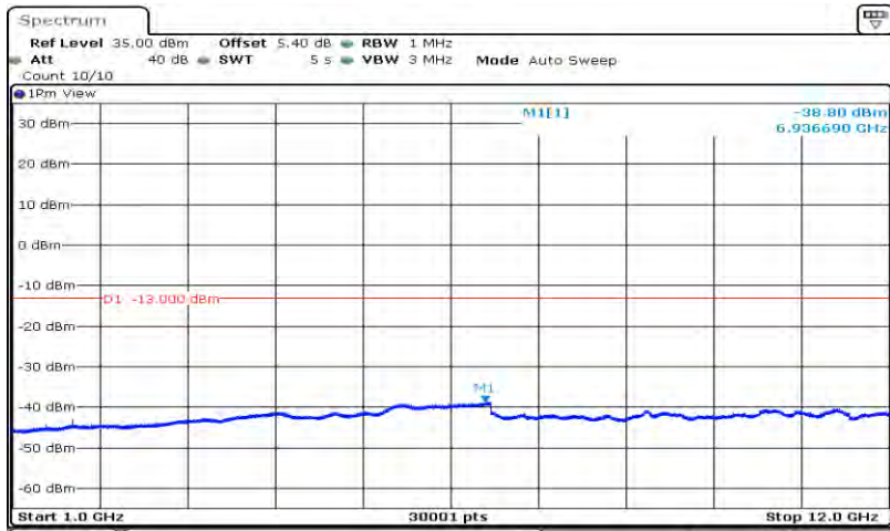
Band12-10MHz-QPSK-23130-1RB#0-Range2:1000~12000MHz
