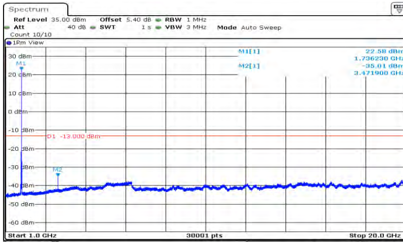
Band4-20MHz-QPSK-20300-1RB#0-Range2:1000~20000MHz
