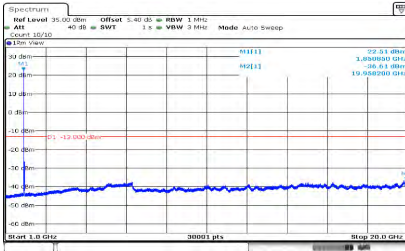
Band2-20MHz-16QAM-18700-1RB#0-Range2:1000~20000MHz
