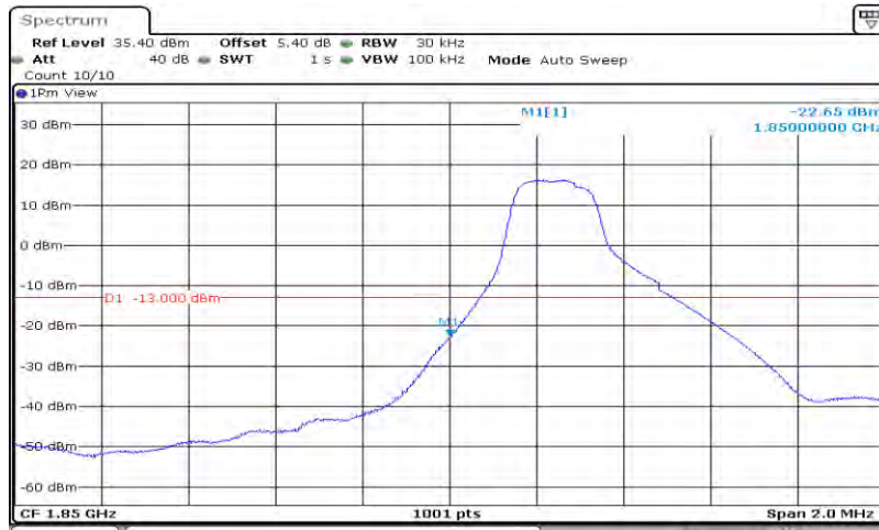
Band2-3MHz-QPSK-18615-15RB#0
