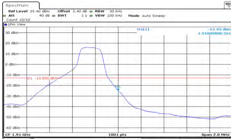
Band2-3MHz-QPSK-19185-15RB#0
