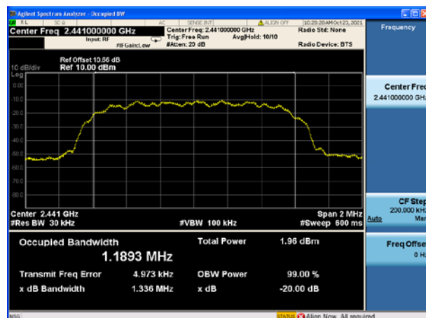
Modulation: \pi/4 DQPSK 2441MHz
