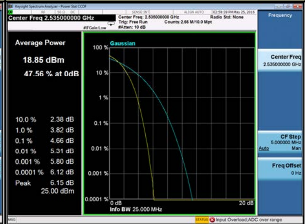
20MHz / 16QAM
