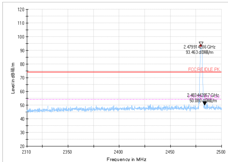
BANEDGE: 8DPSK, Ch78,PK
