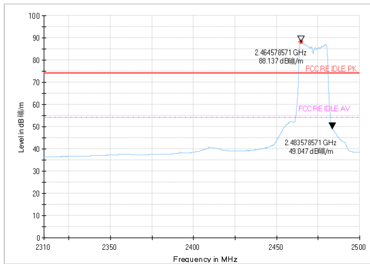
AV detector
