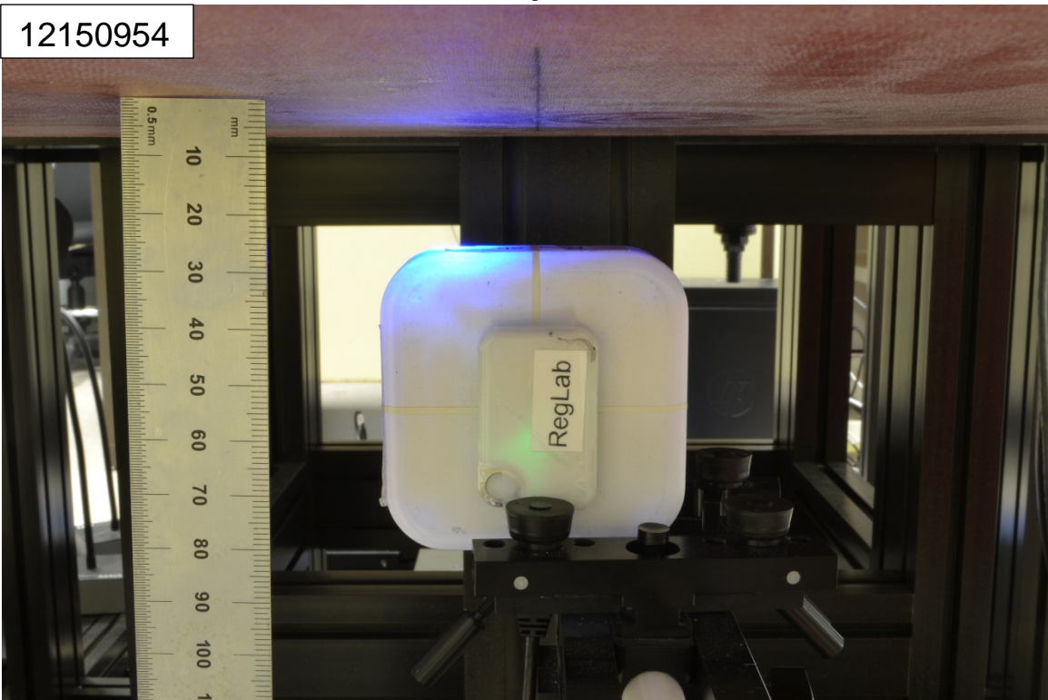
Antenna 1: Edge 1 @25mm
