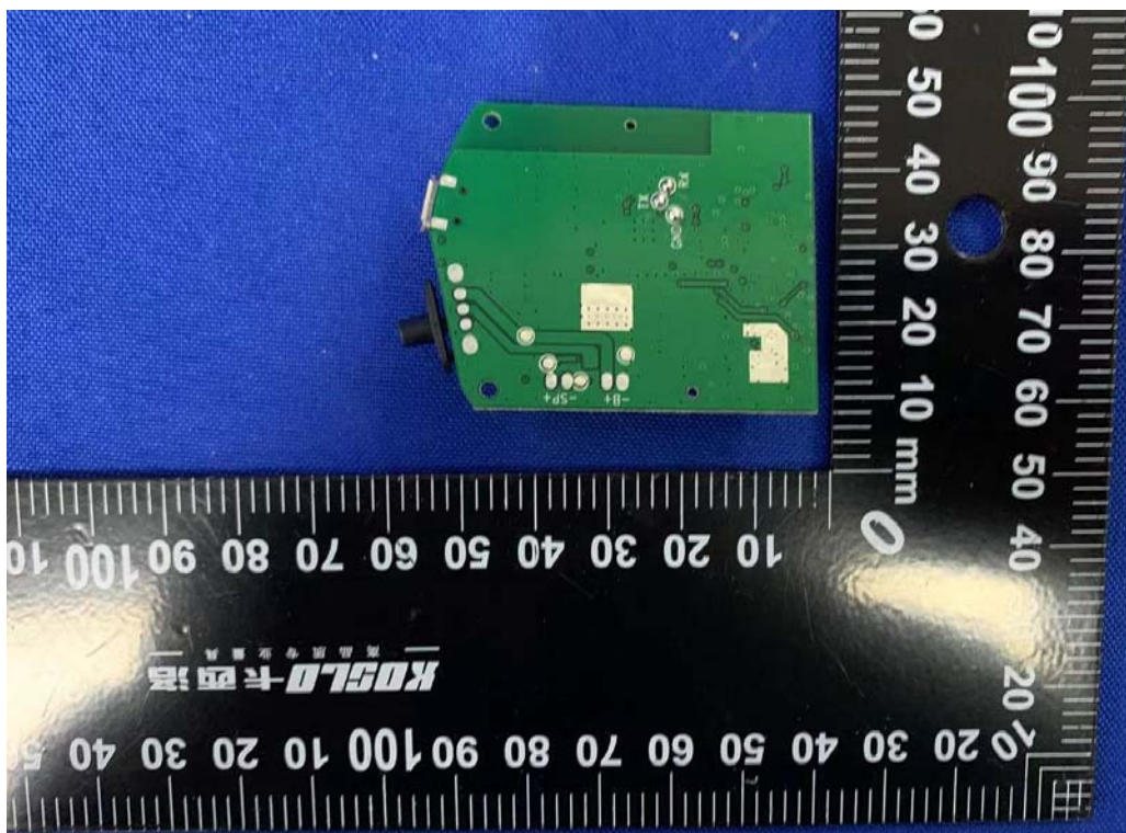
5.8G Antenna
