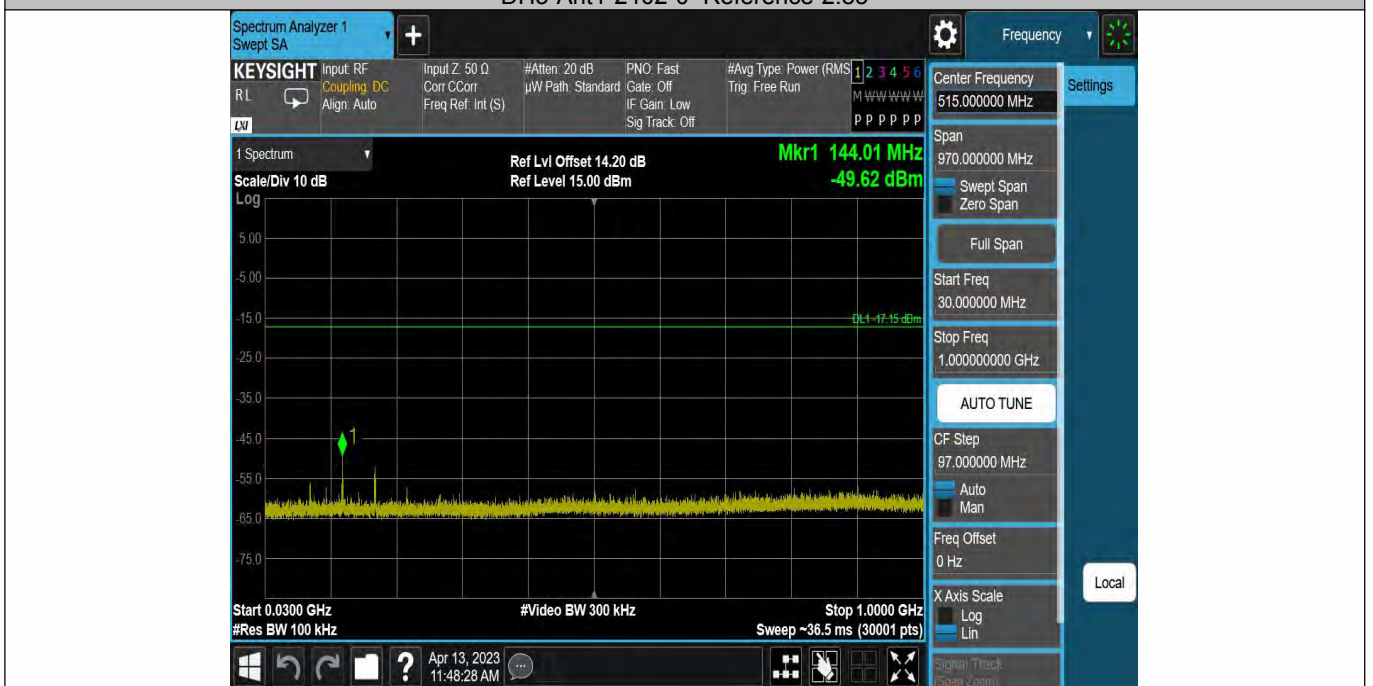
DH5-Ant1-2402-30~1000-2.85
