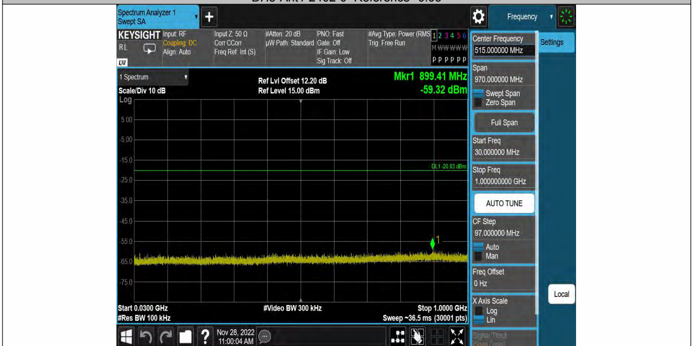
DH5-Ant1-2402-30~1000--0.03
