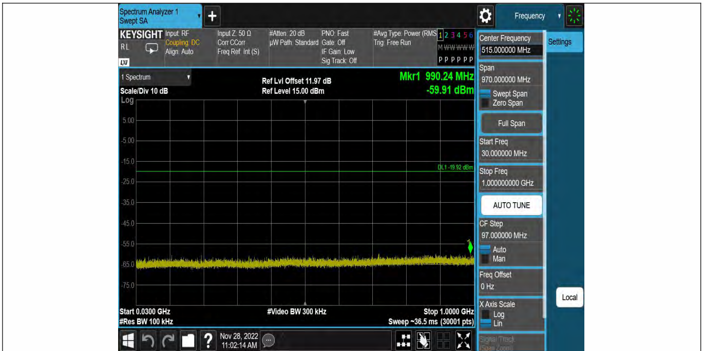
DH5-Ant1-2441-30~1000-0.08
