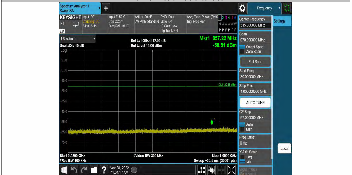
DH5-Ant1-2480-30~1000--0.68
