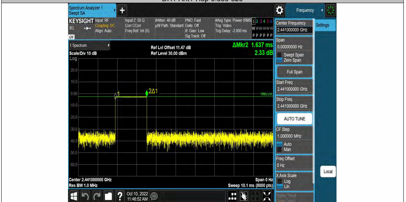
DH3-Ant1-Hop-1.637-160
