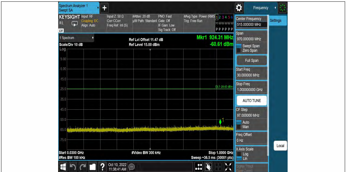
DH5-Ant1-2441-30~1000--4.43
