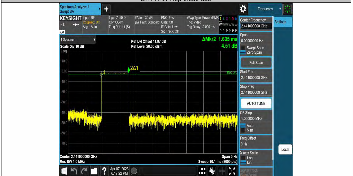
DH3-Ant1-Hop-1.635-160
