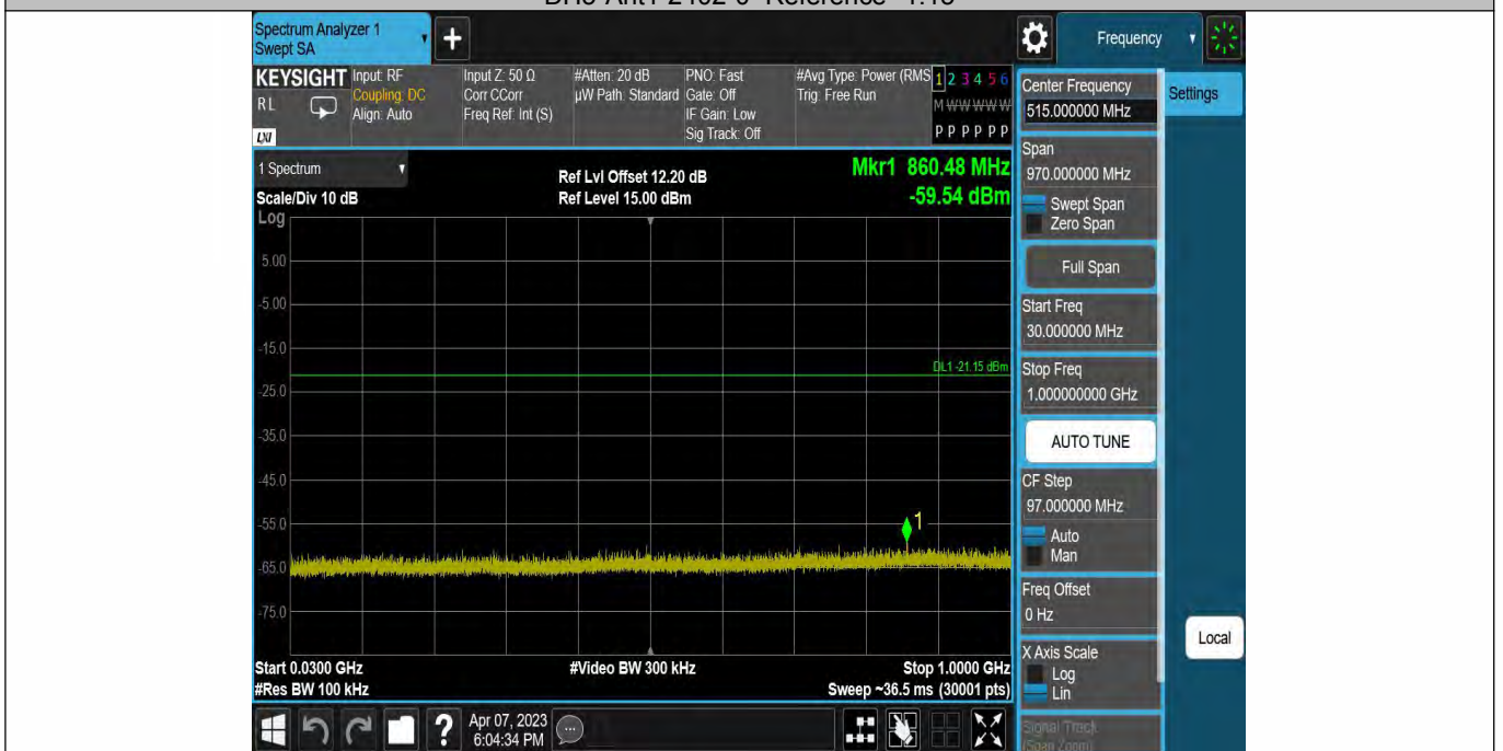
DH5-Ant1-2402-30~1000--1.15
