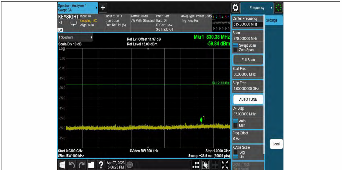
DH5-Ant1-2441-30~1000--1.58
