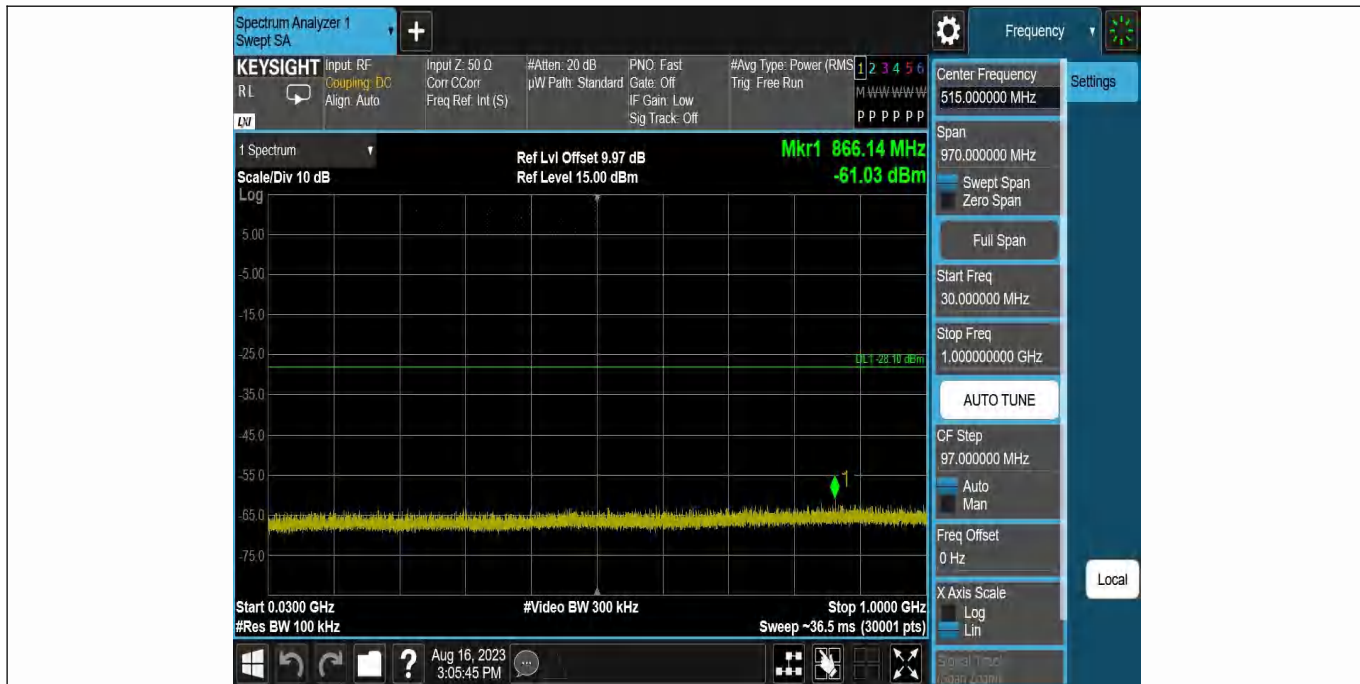
DH5-Ant1-2441-30~1000
