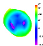
2500.000MHz E1
