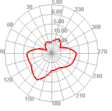
2500.000MHz E1
