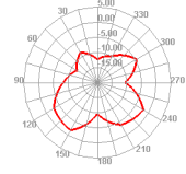
2500.000MHz H
