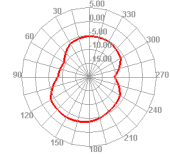
2450.000MHz H
