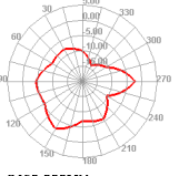
2450.000MHz
