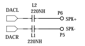
SPK+/-
