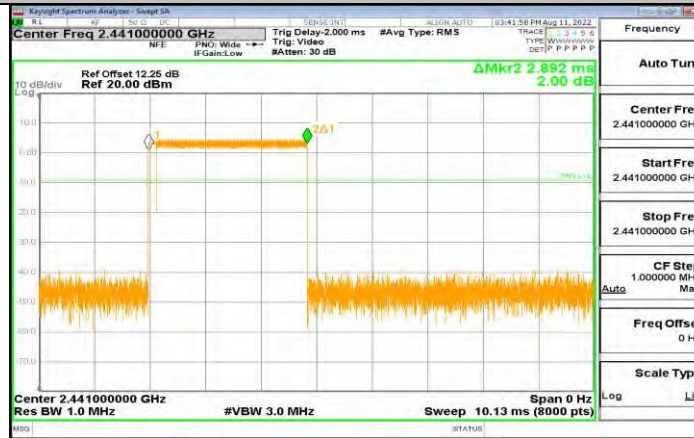
3DH5_Ant1_Hop
