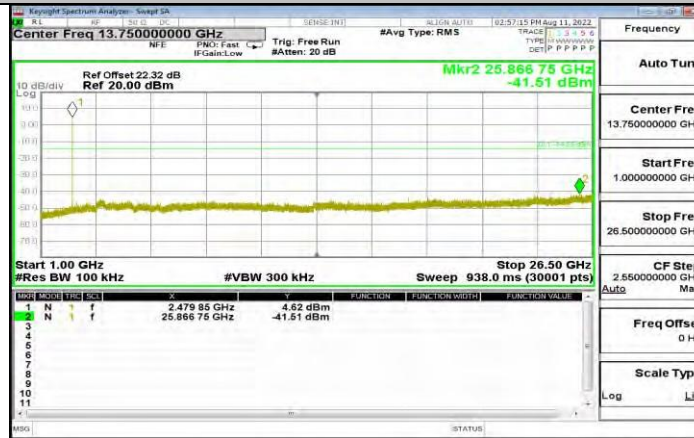
DH5_Ant1_2480_1000~26500
