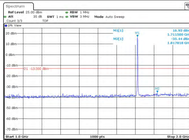
Band4-1.4MHz-QPSK-19957-6RB#0-Range2:1000~2000MHz
