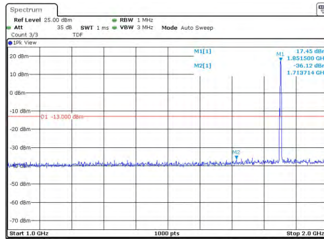
Band2-1.4MHz-QPSK-18607-6RB#0-Range2:1000~2000MHz
