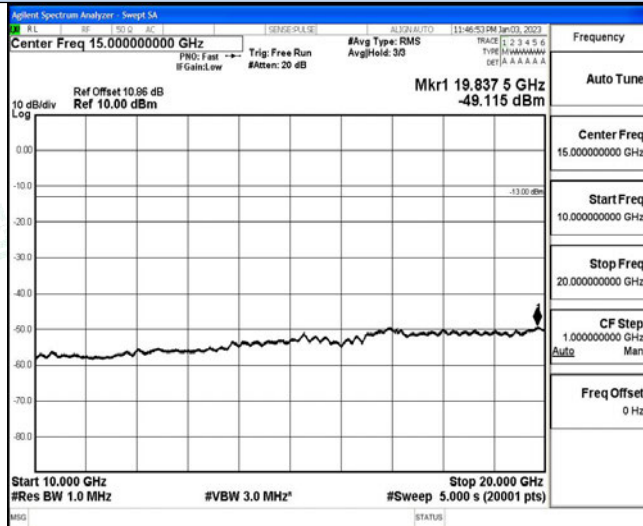
10 GHz – 20 GHz
