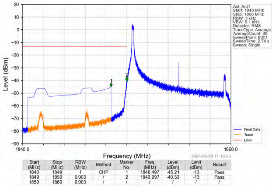
Band25_10MHz_QPSK_LCH_1855MHz_RB_1_0_NTNV
