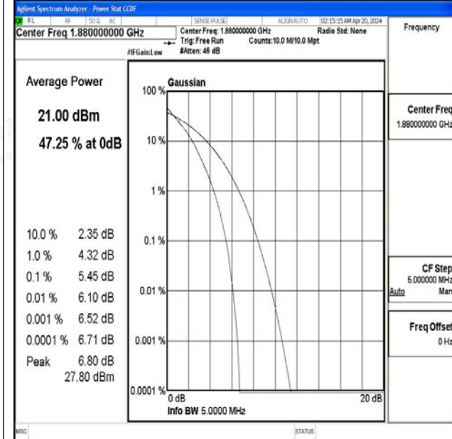
Band2-5MHz-QPSK-18900-25RB#0-PASS
