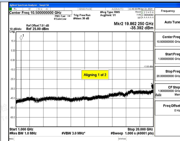
1 GHz – 20 GHz
