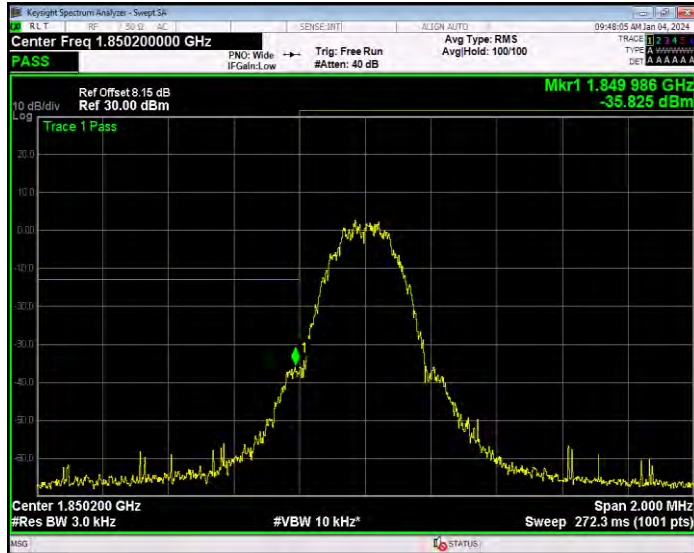
EGPRS1900 Channel=810
