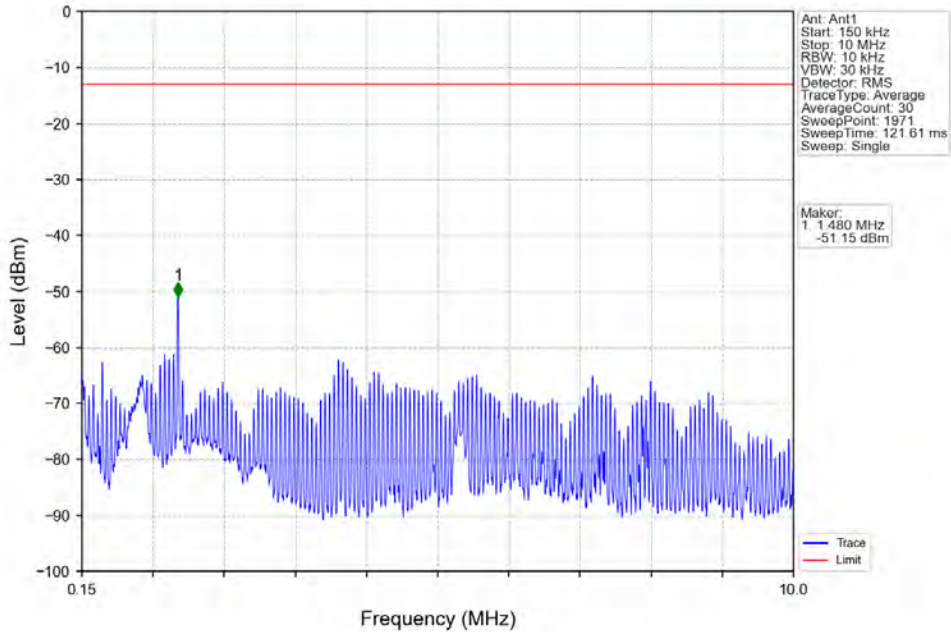
Band66_20MHz_16QAM_LCH_1720MHz_RB_1_0_NTNV
