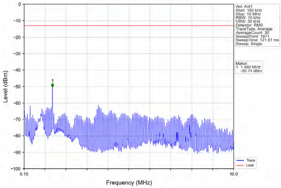
Band66_20MHz_QPSK_MCH_1745MHz_RB_1_0_NTNV
