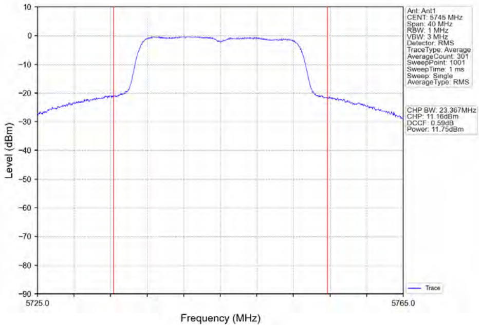
802.11n(HT20)_LCH_5745MHz_Ant1_NTV
