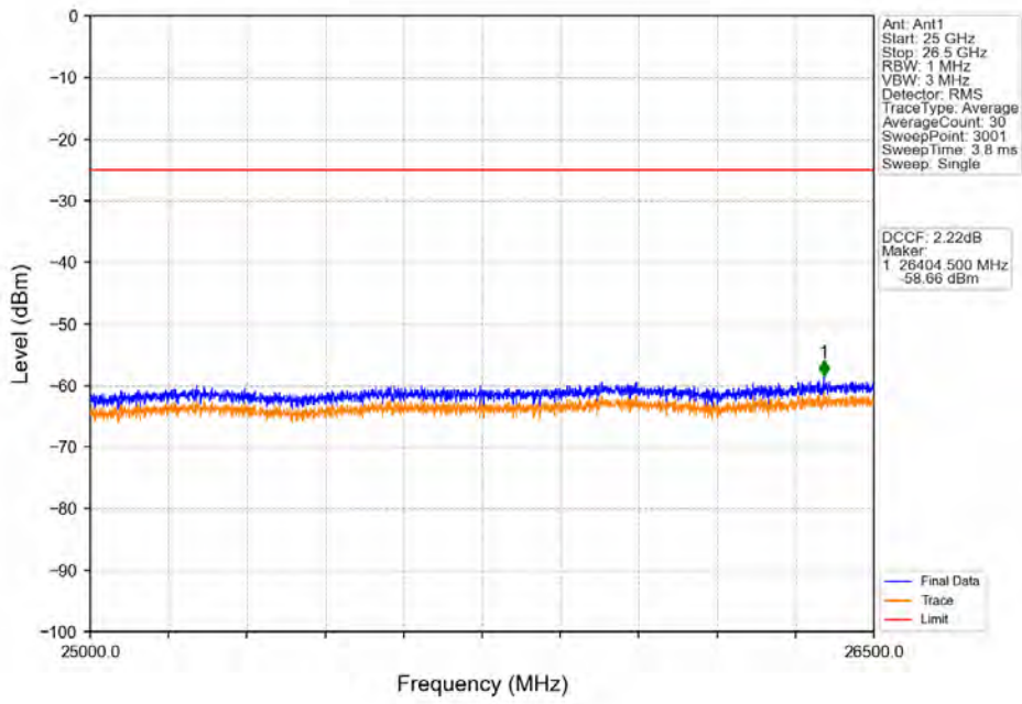
Band41_10MHz_16QAM_LCH_2501MHz_RB_50_0_NTNV
