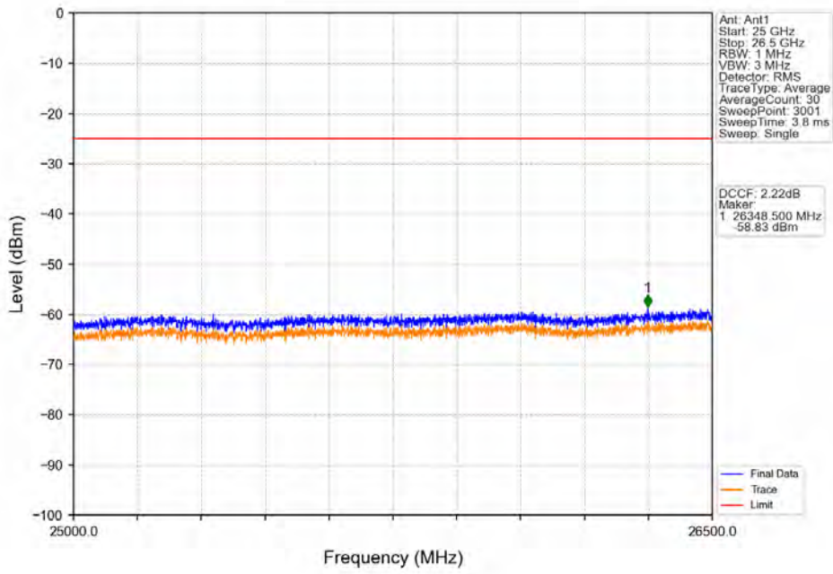
Band41_20MHz_QPSK_HCH_2680MHz_RB_1_99_NTNV
