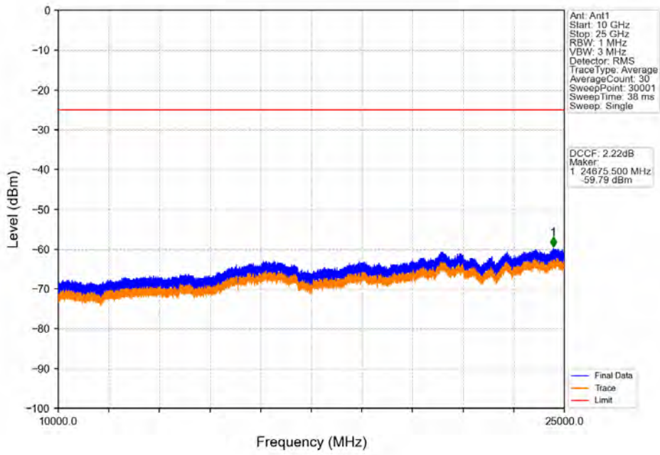
Band41_10MHz_QPSK_LCH_2501MHz_RB_1_0_NTNV
