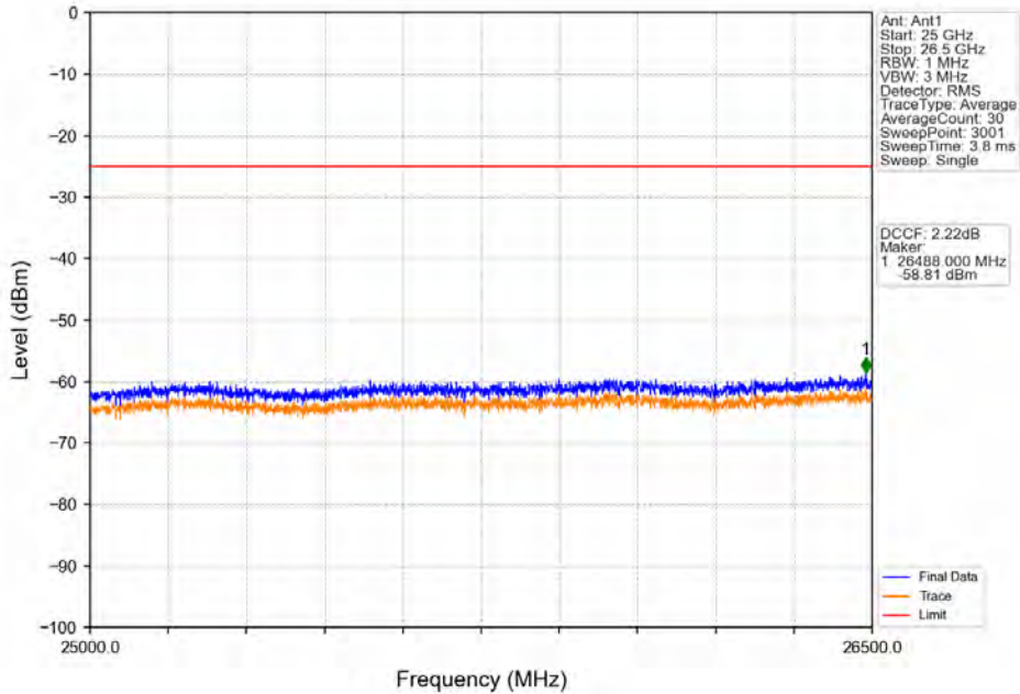
Band41_15MHz_QPSK_LCH_2503.5MHz_RB_1_0_NTNV
