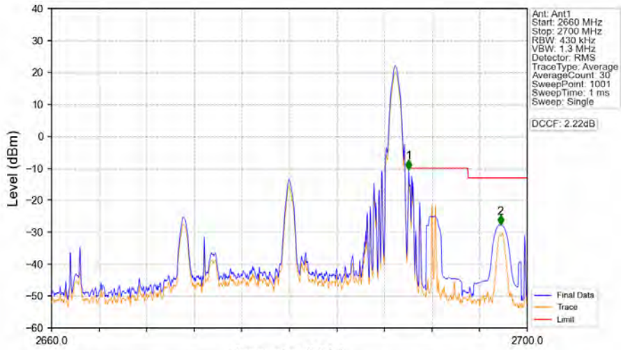
Band41_20MHz_QPSK_HCH_2680MHz_RB_1_99_NTNV
